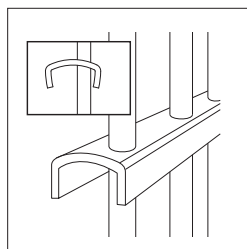
Gepatenteerd U-profiel
